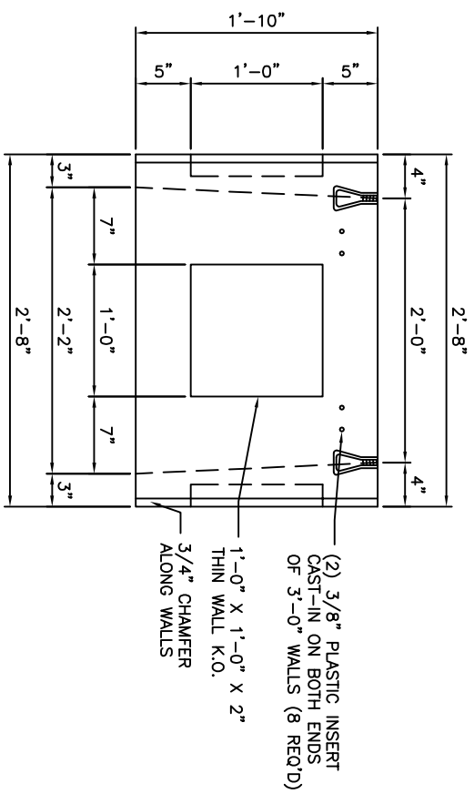
WALL A/C SCALE: 1 1/2" = 1'-0"
